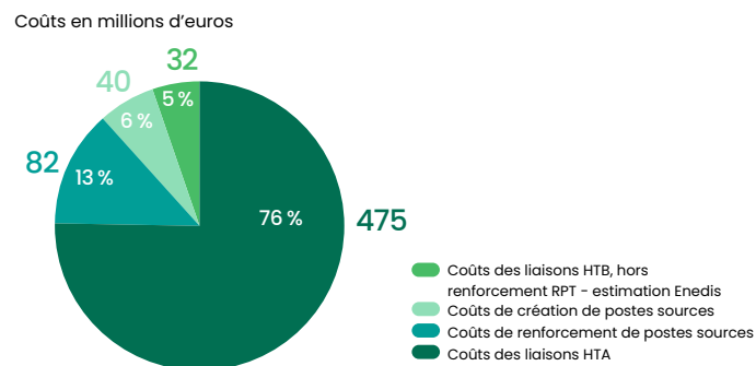
Figure 19 : Répartition des investissements selon la nature des travaux dans le scénario PL BEV haut
